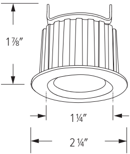
E1AK02 - 1" ROUND DOWNLIGHT
