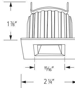
E1AK12 - 1" SQUARE DOWNLIGHT
